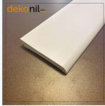
DR10010-D2 10cm Boyanabilir Basic Süpürgelik (100*15*2400mm)
